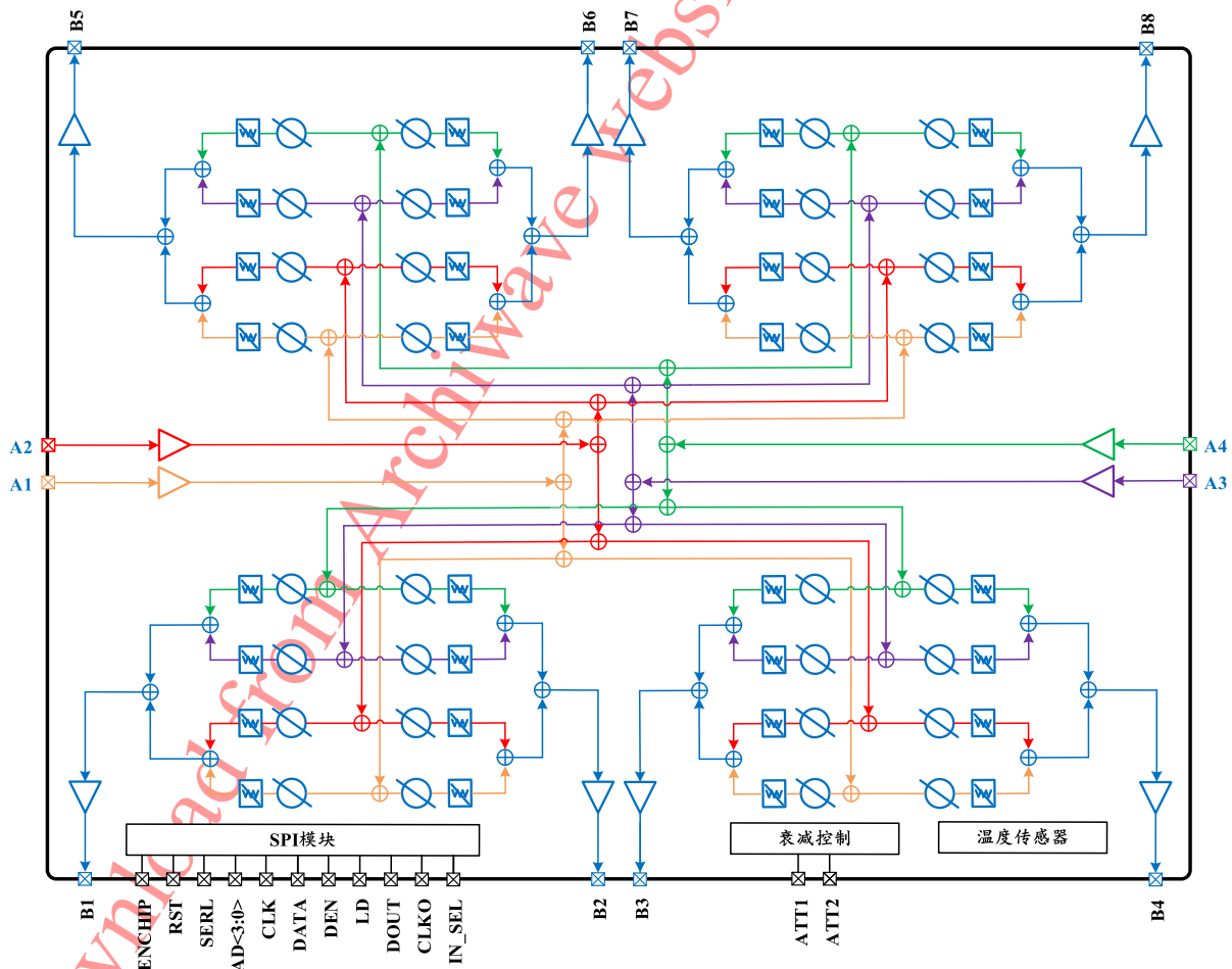
图 1 芯片功能框图
